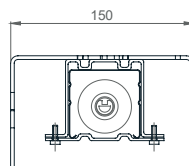
FIX 150 (Einbaumöglichkeit vom Rollo-Insektenschutz)
