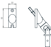
52 X 22mm - 45°
